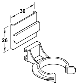
Для накладання
