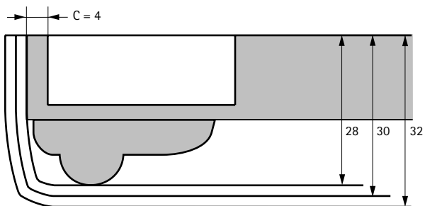
Приклад встановлення мінімальної фуги
