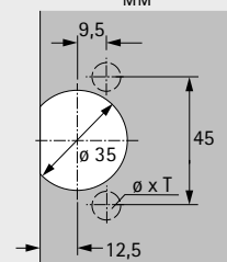
Схема свердління 45 x 9,5 мм
