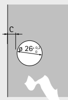
накладна (База В 11 мм)
