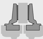
напівнакладна (База В 8 мм)
