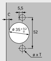
накладна (База В 12.5 мм)
