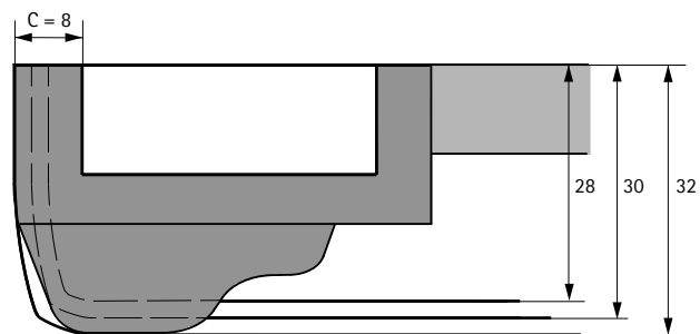
Приклад встановлення мінімальної фуги
