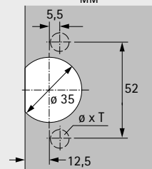
Схема свердління 52 x 5,5 мм
