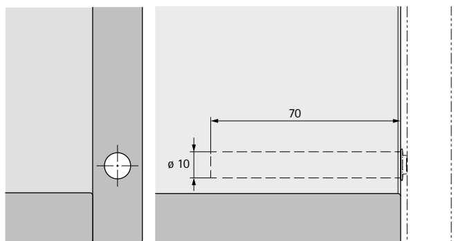
Схема свердління для довгого ходу, для накладних дверей
