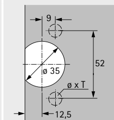
Схема свердління 52 x 9 мм
