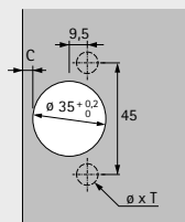
накладна (База В 6 мм)
