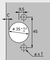
накладна (База В 26 мм)
