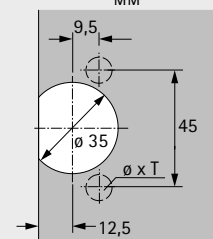
Схема свердління 45 x 9,5 мм
