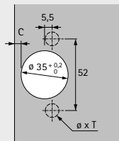
накладна (База В 9 мм)
