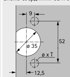
Схема свердління 52 x 9 мм
