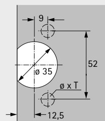
Схема свердління 52 x 9 мм
