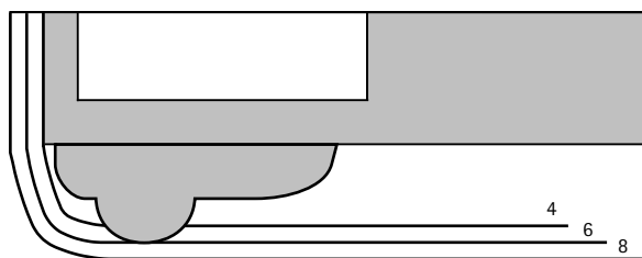
Приклад встановлення мінімальної фуги
