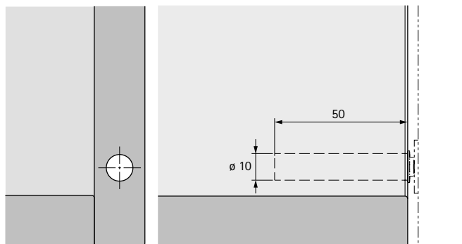
Схема свердління для короткого ходу, для накладних дверей
