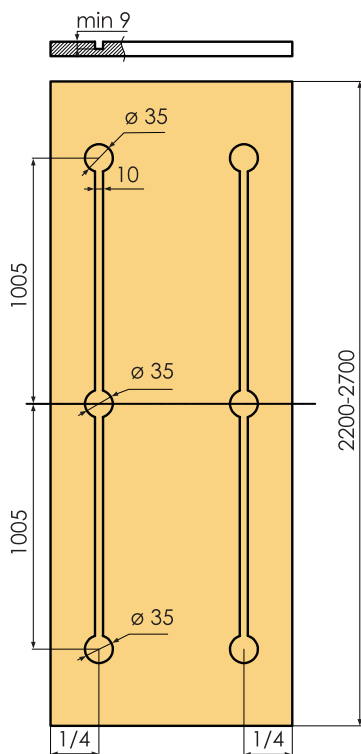
Schemat rozmieszczenia otworów montażowych "A"
