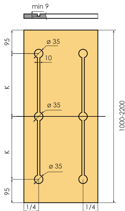
Schemat rozmieszczenia otworów montażowych "A"
