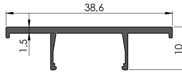
Zaślepka dekoracyjna na profil pionowy (uchwyt)
