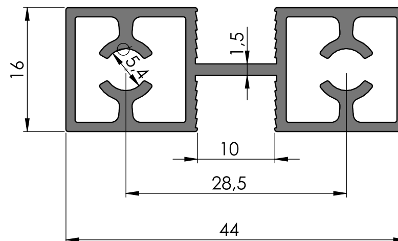
Profil łączący wpuszczany
