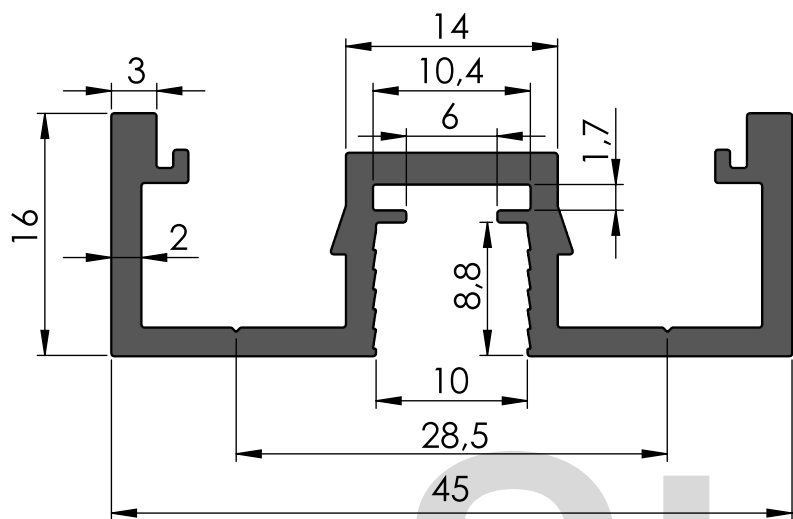
Profil pionowy (uchwyt)
