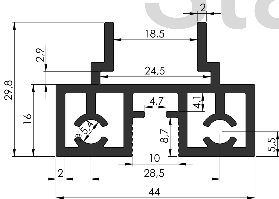
Profil poziomy (uniwersalny)
