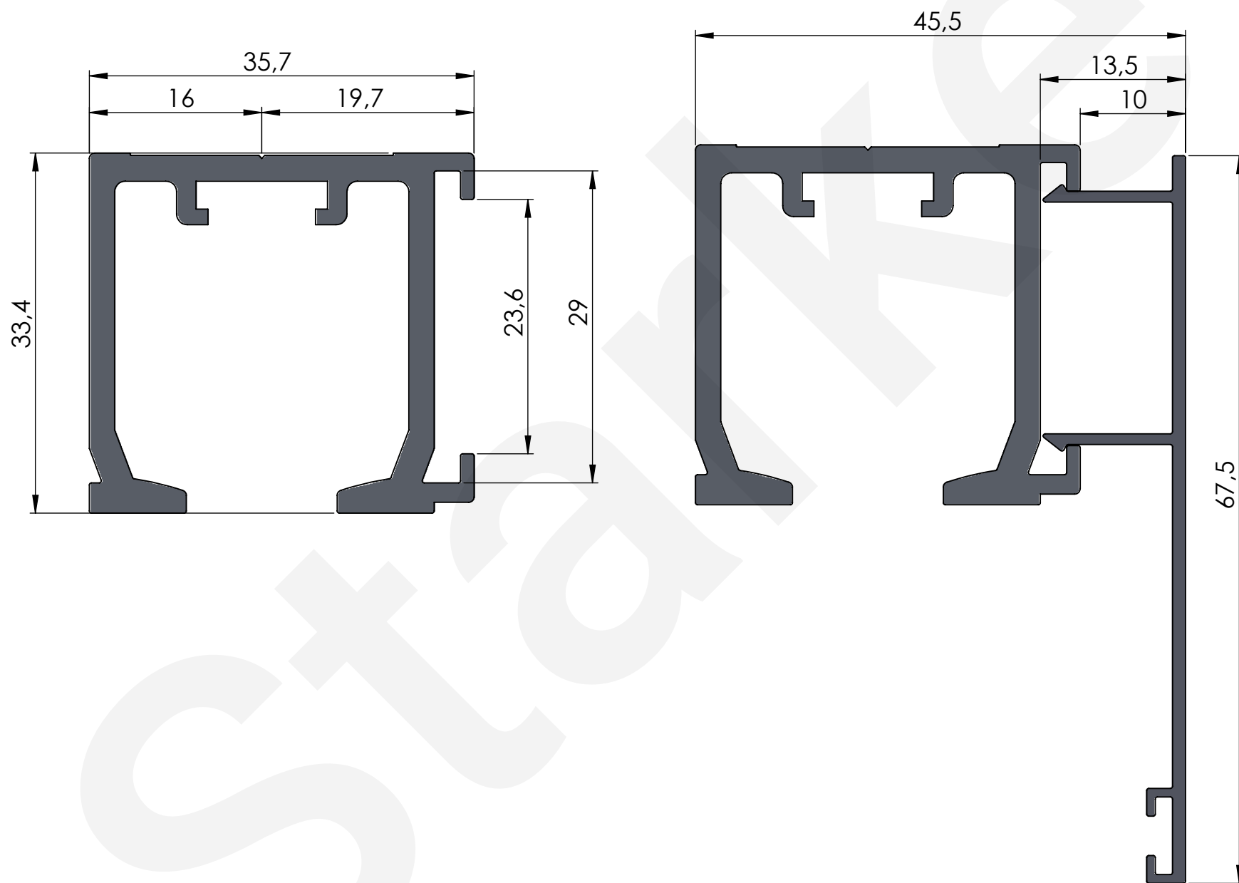
Rysunek techniczny prowadnicy do ścianki działowej Starke
