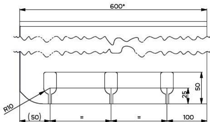
Рекомендована схема фрезерування (для жорсткішого з'єднання)
