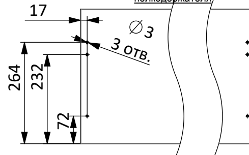
Сверловка фасада для установки полкодержателя
