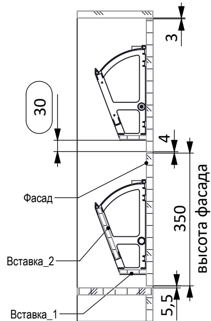
Сверловка фасада для установки полкодержателя
