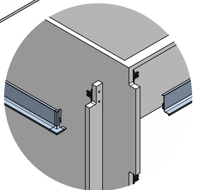
DETTAGLIO A
