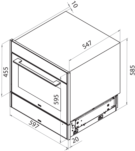
Креслення монтажу із шафою для підігріву посуду
