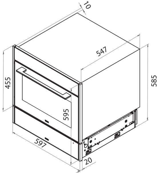
Креслення монтажу із шафою для підігріву посуду
