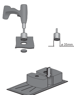
Монтаж мийок Franke у рівень зі стільницею
