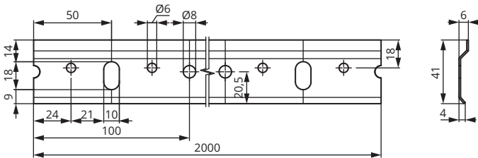
Вушко для навішування шаф оцинковане
