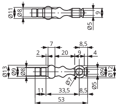
Стовпчик-кріплення релінга, кінцеве
