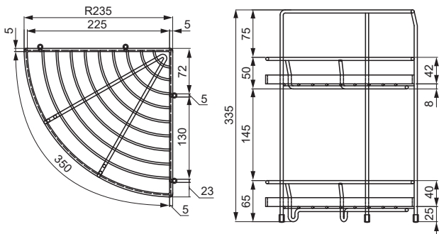
Підставка під гаряче
