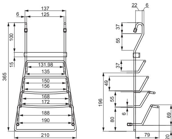
Полиця кутова (подвійна)
