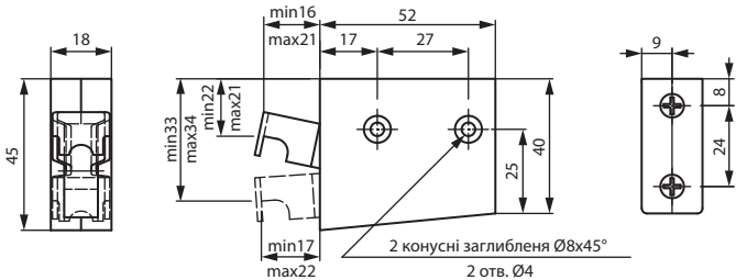
Вушко регульоване універсальне
