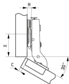
Арт. № 12700 Кут +30°
