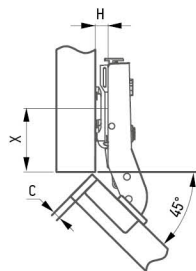
Арт. № 12699 Кут +45°
