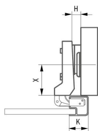
Арт. № 25388 ЗАВІСА НАПІВНАКЛАДНА
