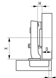
Арт. № 97744 ЗАВІСА НАКЛАДНА
