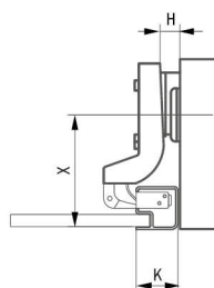
Арт. № 25389 ЗАВІСА ВНУТРІШНЯ
