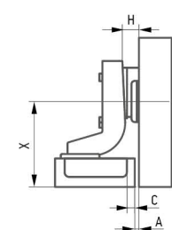
Арт. № 97745 ЗАВІСА ВНУТРІШНЯ
