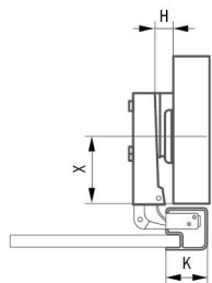
Арт. № 25387 ЗАВІСА НАКЛАДНА
