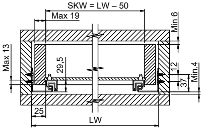
Монтажні розміри
