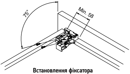
Встановлення фіксатора
