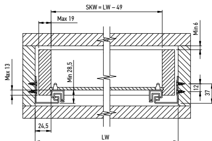
Монтажні розміри
