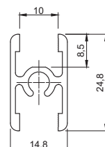
Профиль с приливом
