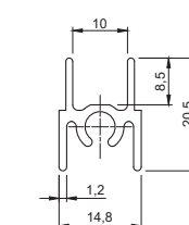
Профиль горизонтальный верхний
