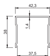
Верхняя рельса одинарная
