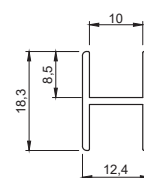
Профиль H-образный
