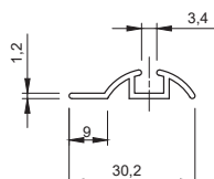
Нижняя рельса одинарная
