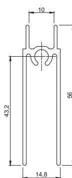
Профиль горизонтальный нижний
