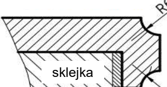
kraw. opadająca z wklęsłą fazką R6+R6
