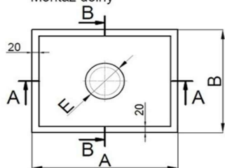
Umywalka WSF09 (Zmienne wymiary w milimetrach)
