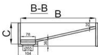
Umywalka WS04 (Zmienne wymiary w milimetrach)
