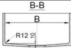
Zlewozmywak SS04 (Zwane wymiary w milimetrach)
