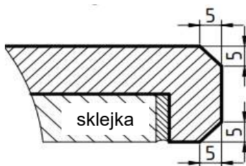
kraw. opadająca z fazką 5x5+5x5
