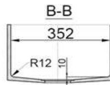
Zlewozmywak SR06 (Zmienne wymiary w milimetrach)
