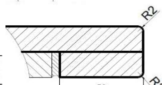
kraw. opadająca R2xR2 podwinięcie
