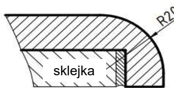
kraw. opadająca z fazką R20
