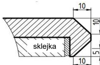
kraw. opadająca z fazką 10x10
