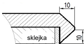
kraw. opadająca 10x10x10+10x10
