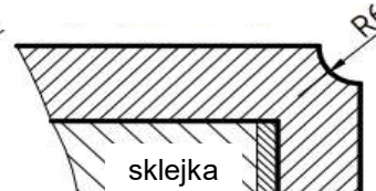
kraw. opadająca z wklęsłą fazką R6
