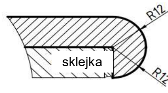
kraw. opadająca z fazką R12+R12
