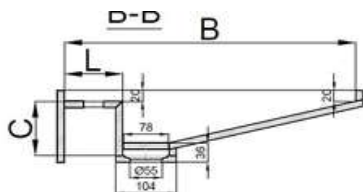
Umywalka WS03 (Zmienne wymiary w milimetrach)
