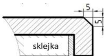
kraw. opadająca 5x5
