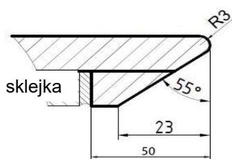
kraw. opadająca R3 (SharkNose 55)
