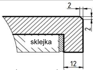
kraw. opadająca z fazką 2x2
