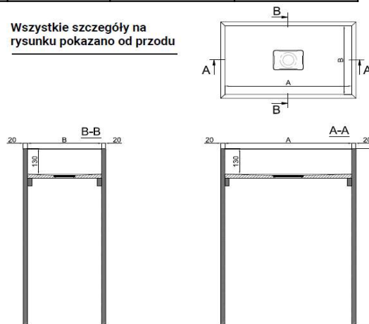
ZMIENNE WYMIARY (MM)
