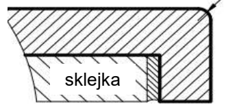
kraw. opadająca z fazką R3
