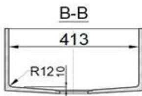
Zlewozmywak SS03 (Zwane wymiary w milimetrach)
