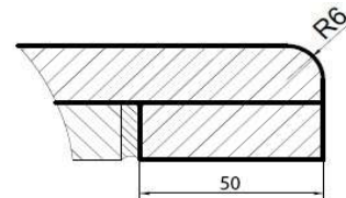
kraw. opadająca R6 podwinięcie
