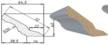
Карниз Лоренцо прямий
