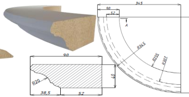
Карниз Лоренцо радіусний
