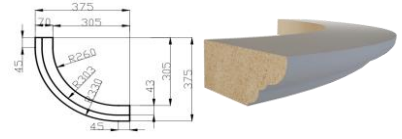
Карниз складний радіусний
